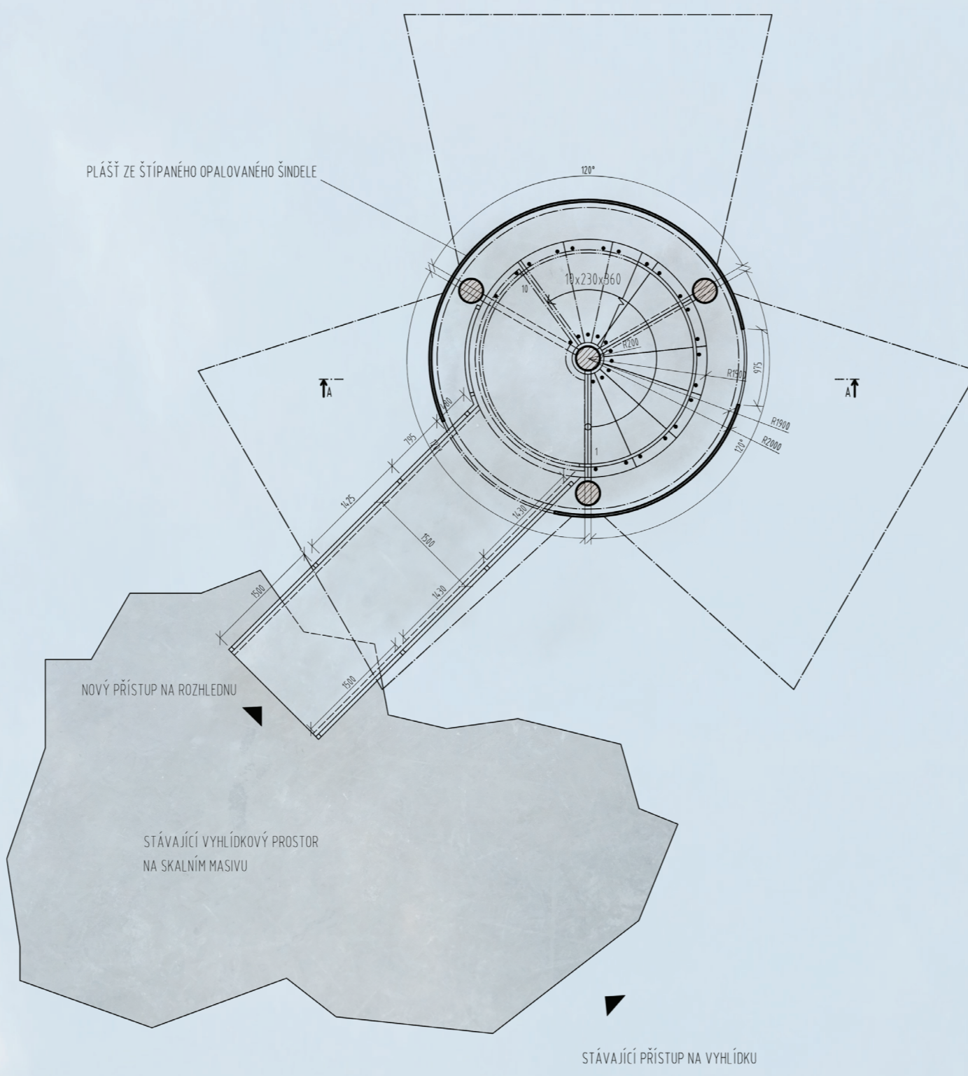
KONSTRUKČNÍ SCHEMA
