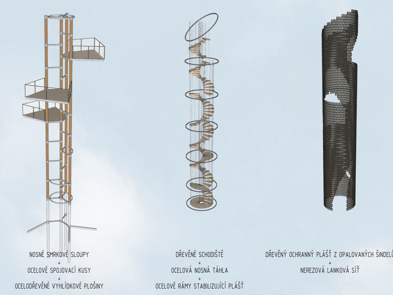
KONSTRUKČNÍ SCHEMA
