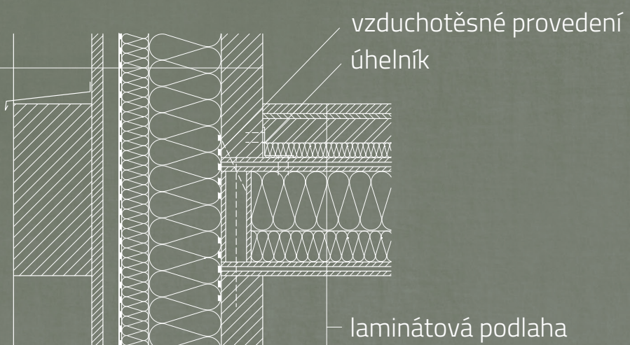
konstrukční detail spoj stropní a obvodové konstrukce
