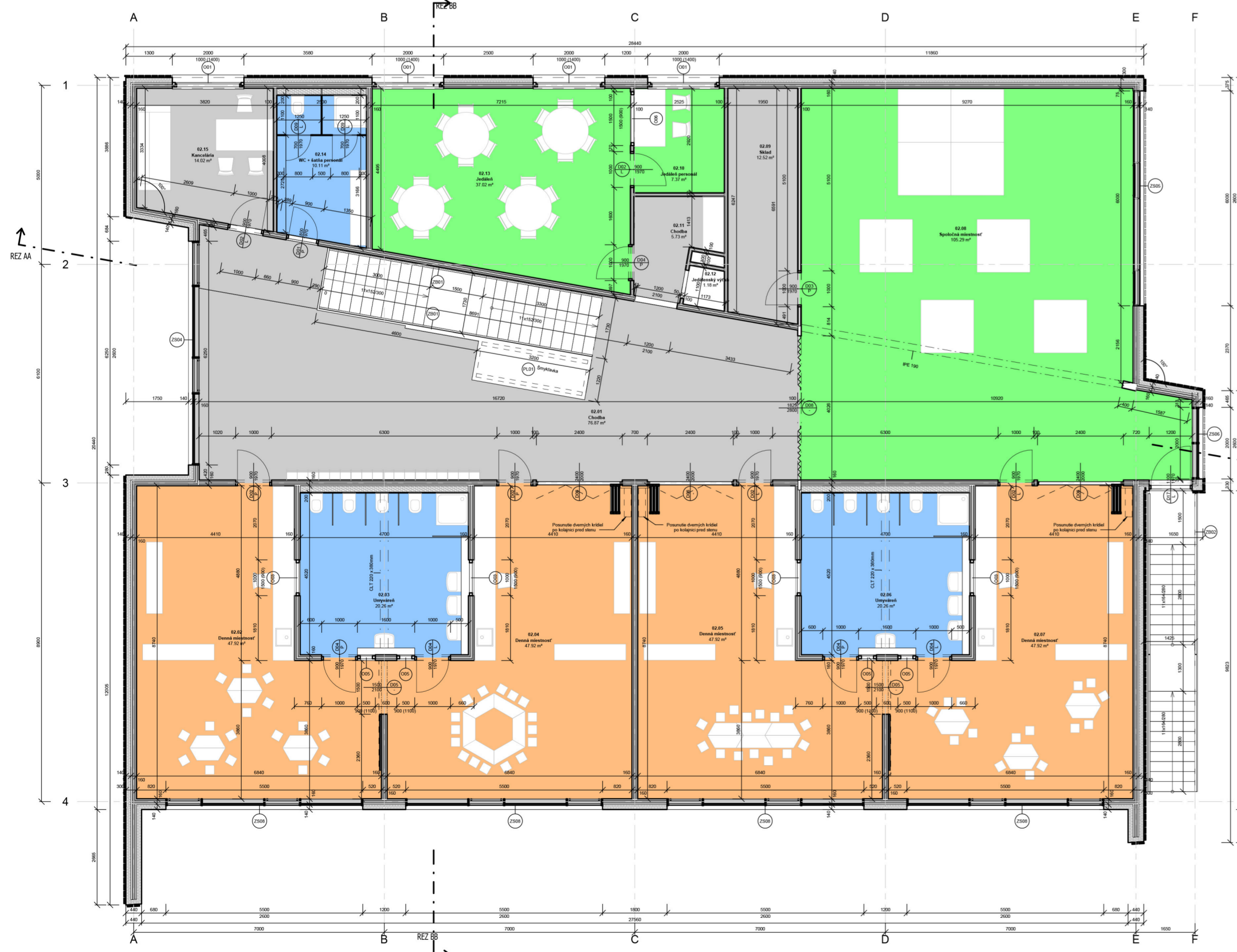
Pódorys 2.NP
