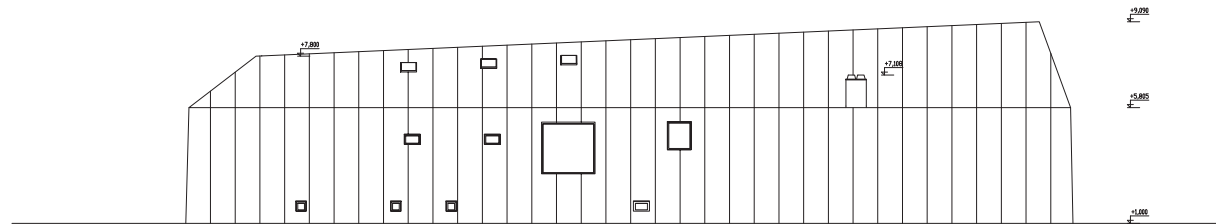
SEVERNÍ POHLED 1:200
