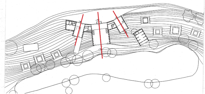
Rezy 1:200 Tri rezy hlavnými priestormi, Kaviareň, Prednášková hala, Výukové centrum (podložené pôdorysom)
