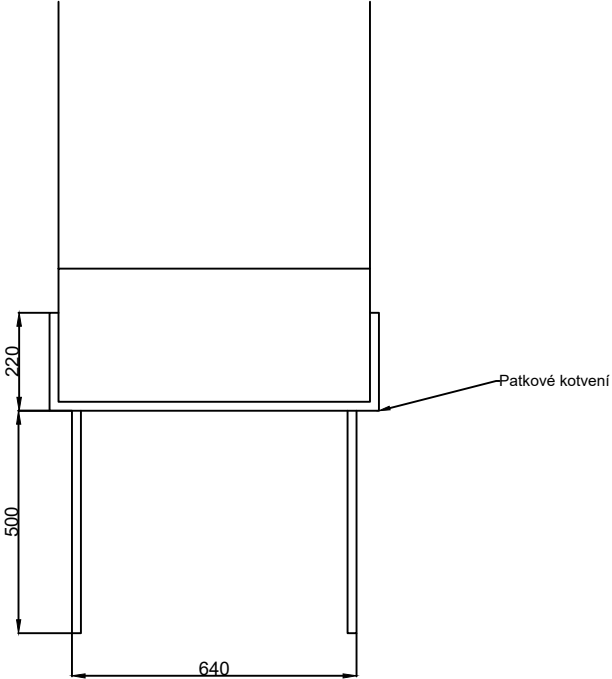
Ukotvení rámu do země
