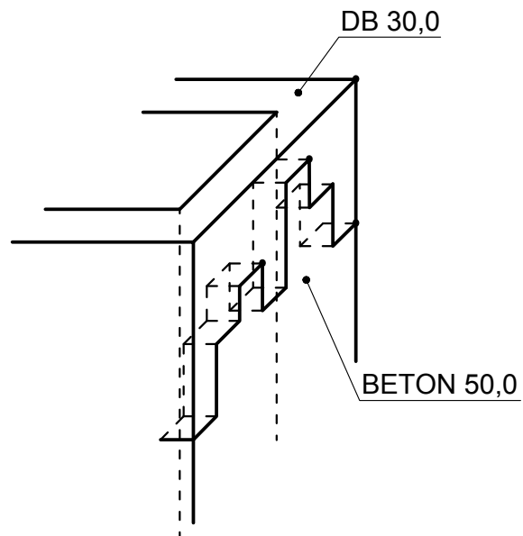
DETAIL Č.3
