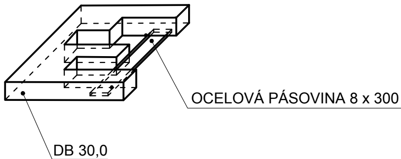
DETAIL Č.1
