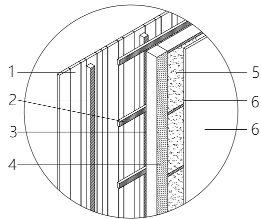
AXONOMETRIA
