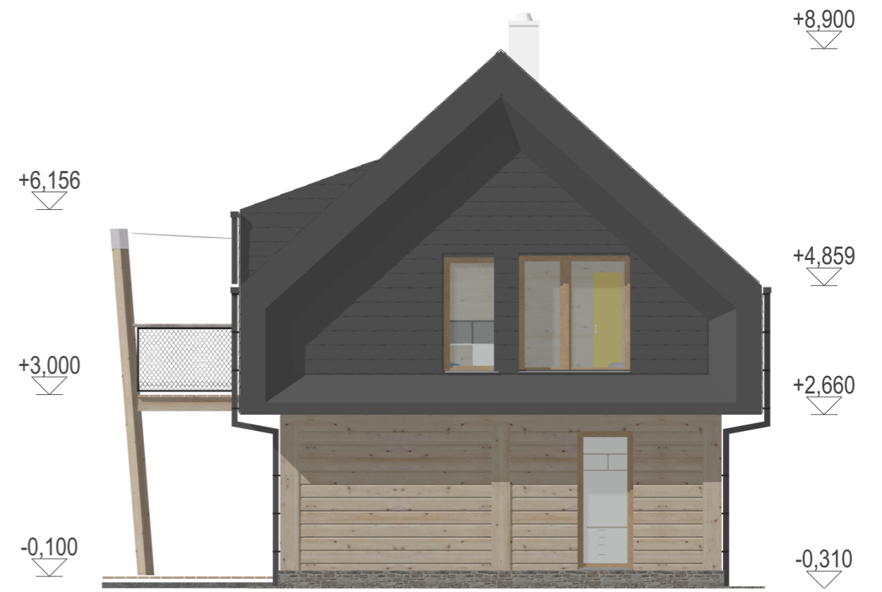
pohled východní
