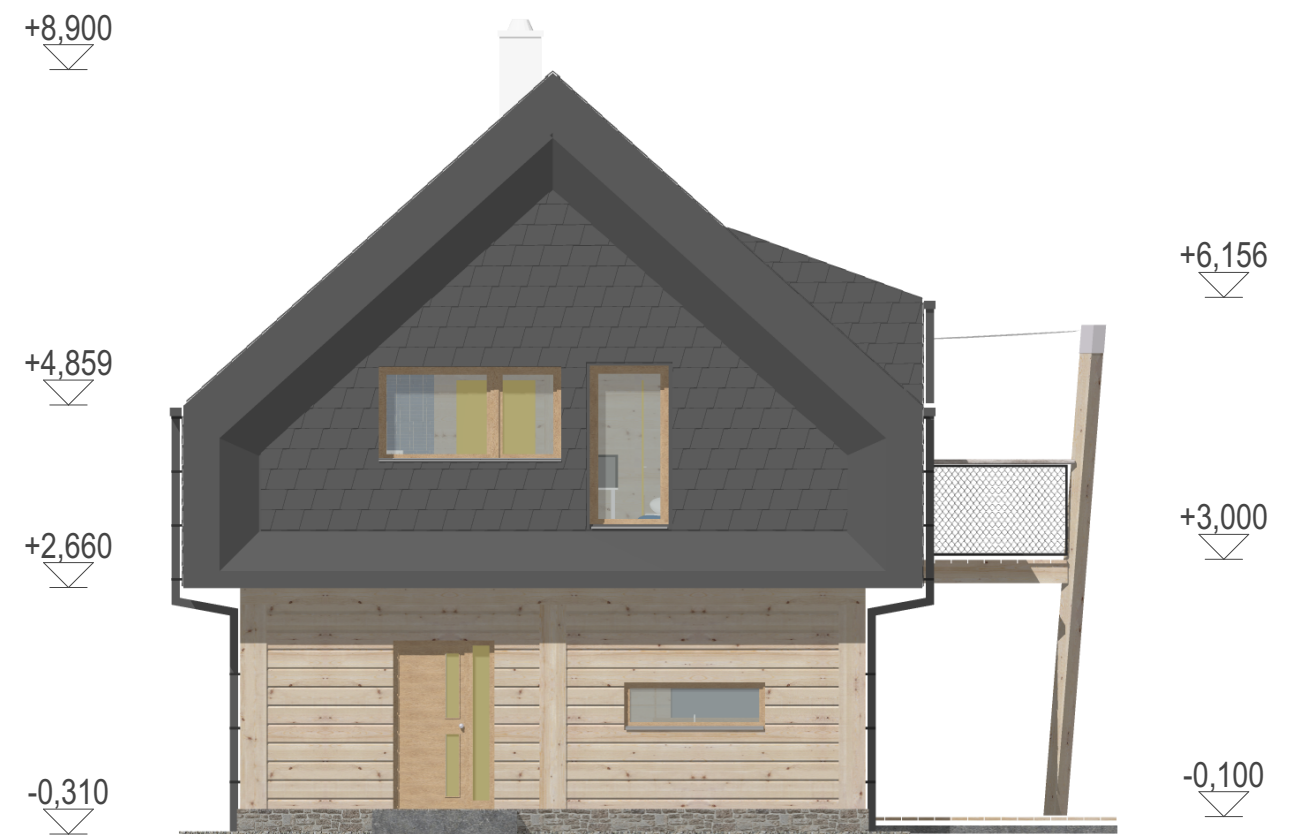
pohled západní
