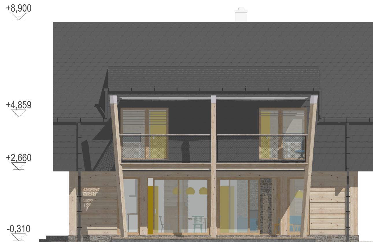
pohled jižní
