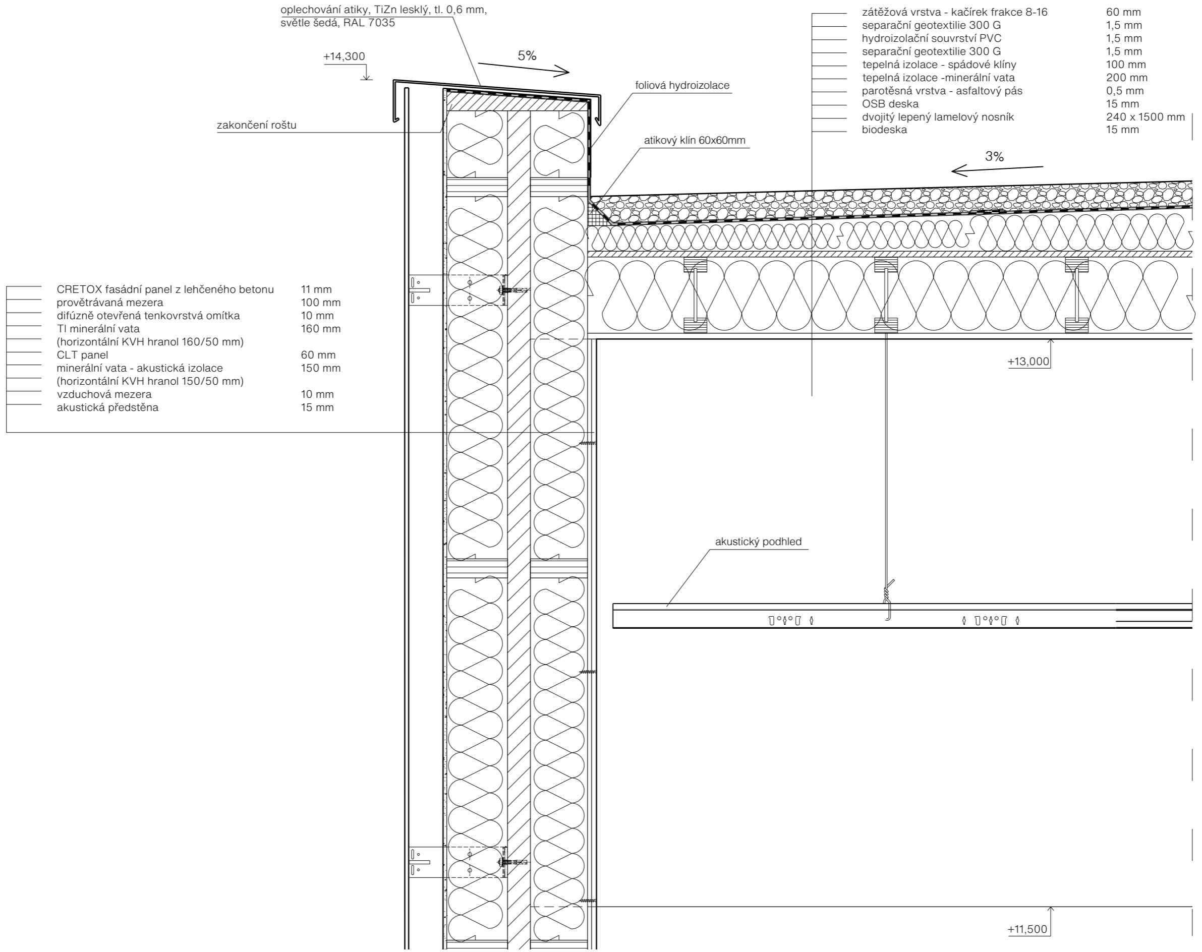
detail D I stavební část
