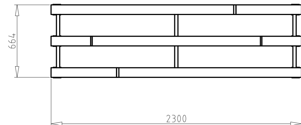
Přodorys
