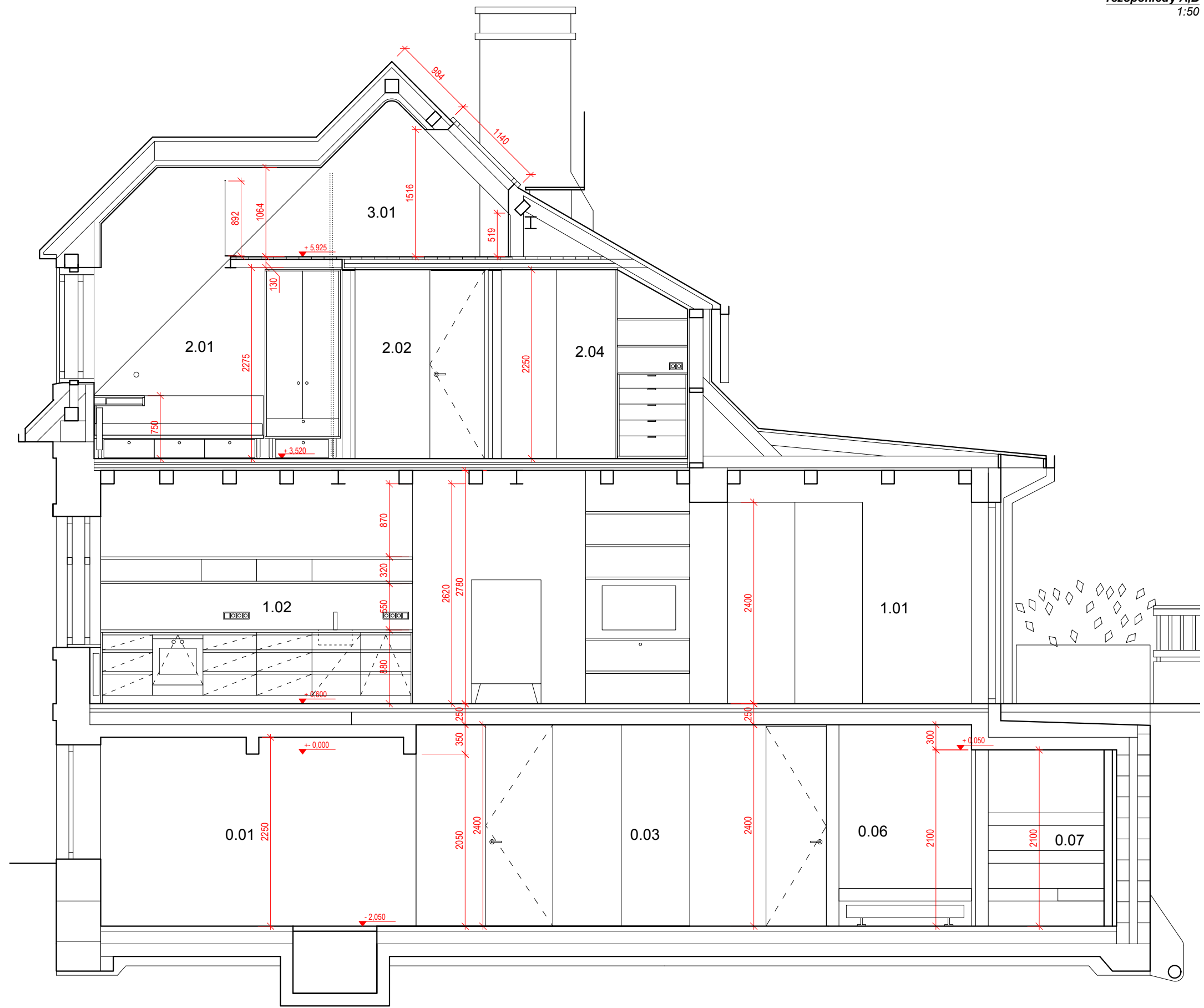
PODÉLNÝ ŘEZ B
